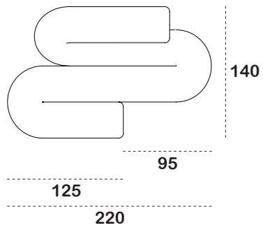
SR 220 C1
