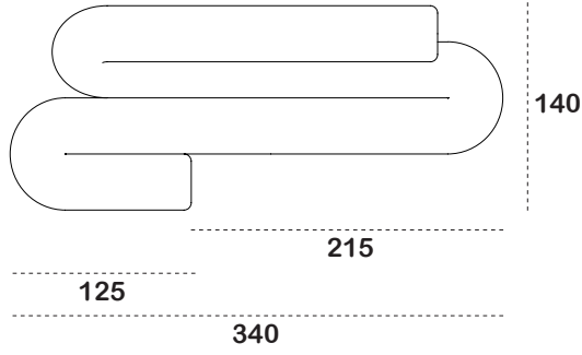
SR 340 C1
