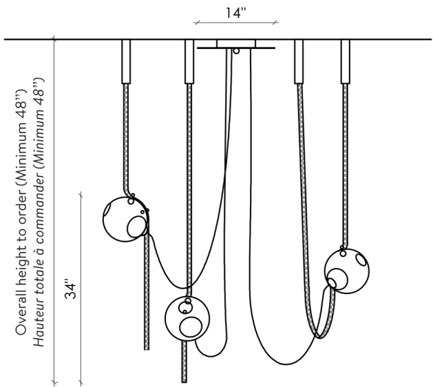
FRONT VIEW VUE DE FACE
