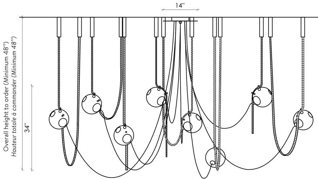
FRONT VIEW VUE DE FACE
