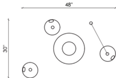
TOP VIEW VUE DE DESSUS
