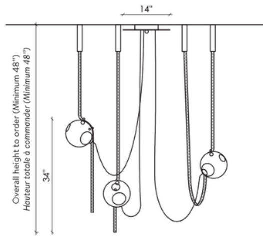
FRONT VIEW VUE DE FACE
